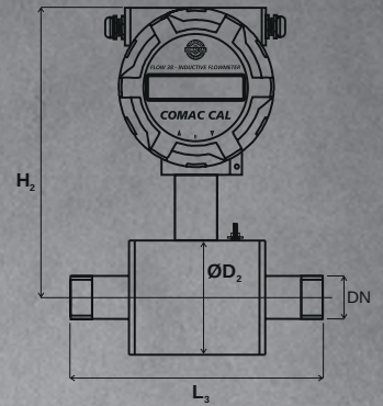
THREAD (EN 10226-1)
